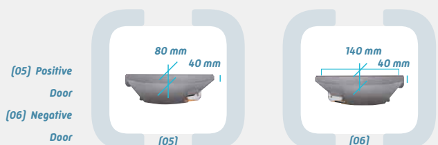
Pivot Door
