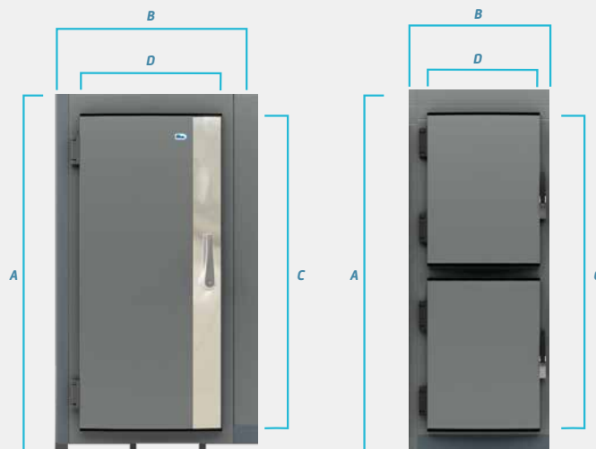
Puertas Pivotantes
