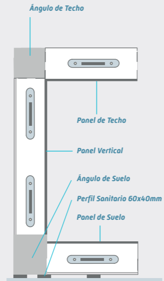
MATRIX 60, 85 e 105 - CON SUELO
