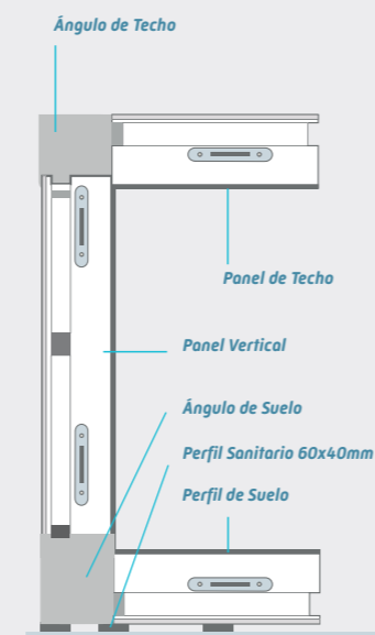
MATRIX 150 - CON SUELO
