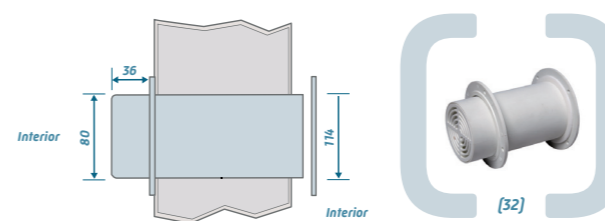
(32) Válvula de Balance de Presión T2-21
