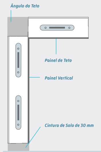
MATRIX 60, 85 e 105 - SEM SOLO
