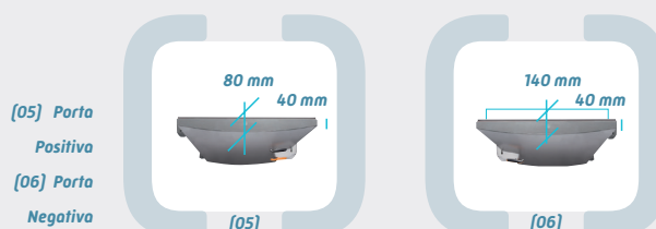
Porta Pivotante
